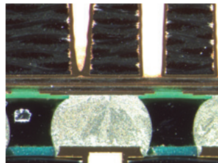
M205C:スルーホール
