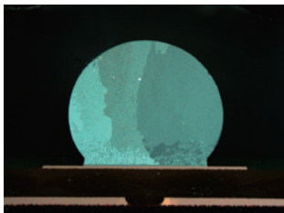
RM2265:ハンダポンプ偏光観察
